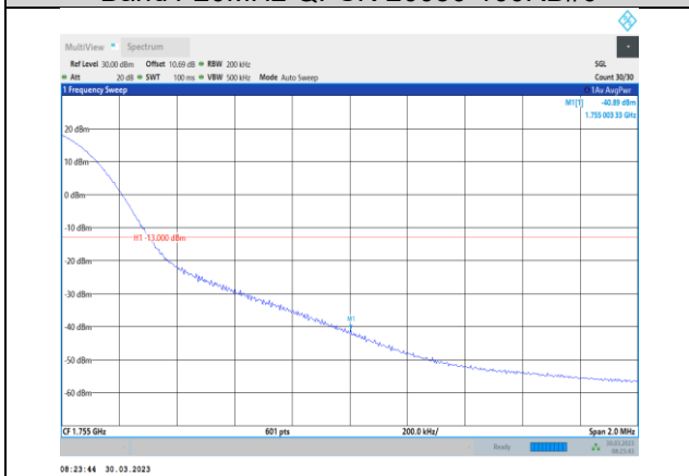
Band4-20MHz-QPSK-20300-1RB#99
