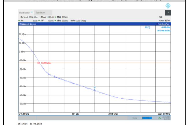
Band2-20MHz-64QAM-19100-1RB#99
