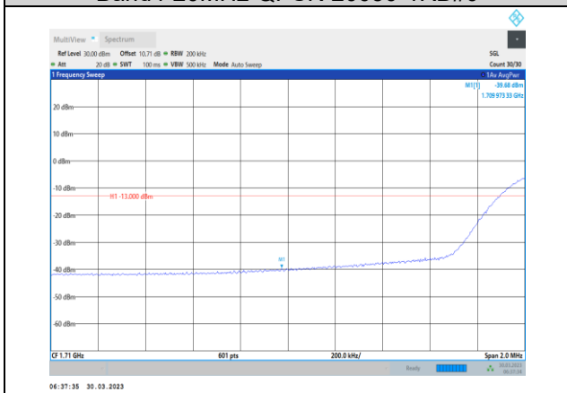
Band4-20MHz-QPSK-20050-100RB#0
