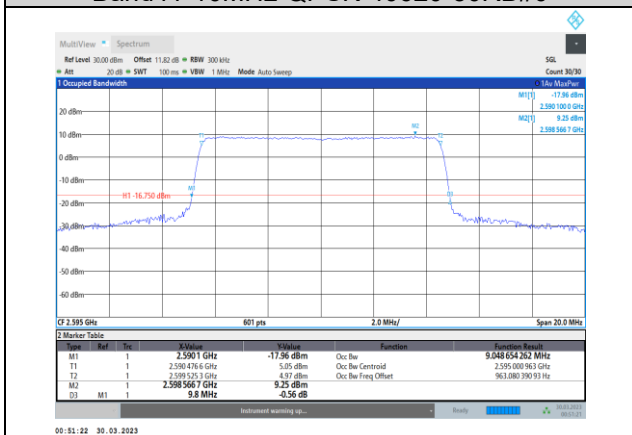
Band41-10MHz-QPSK-40640-50RB#0
