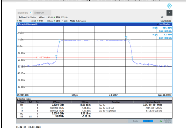
Band41-10MHz-QPSK-40740-50RB#0
