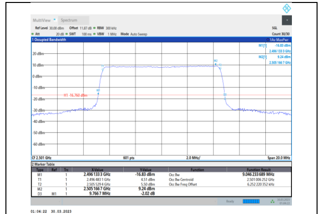
Band41-10MHz-QPSK-39700-50RB#0
