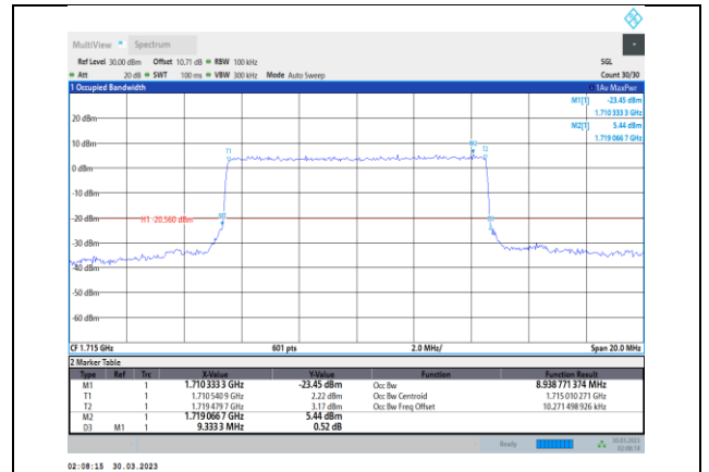
Band4-10MHz-QPSK-20000-50RB#0
