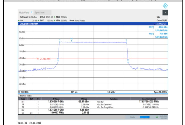
Band2-20MHz-QPSK-18900-100RB#0
