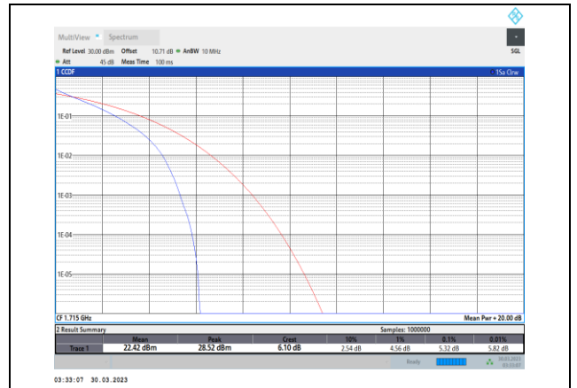
Band4-10MHz-QPSK-20000-50RB#0
