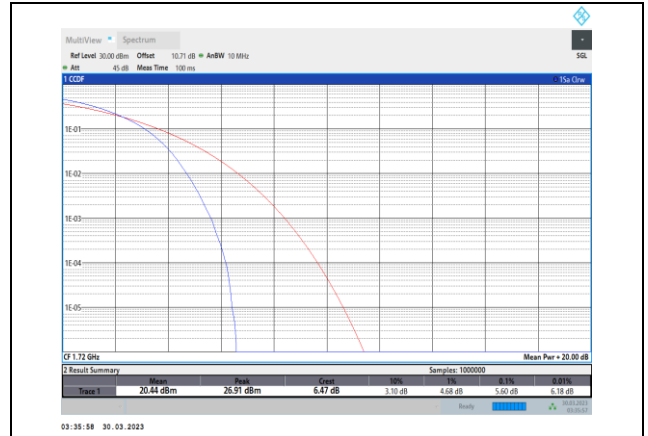
Band4-20MHz-QPSK-20050-100RB#0
