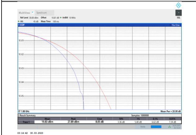
Band2-20MHz-16QAM-18900-100RB#0
