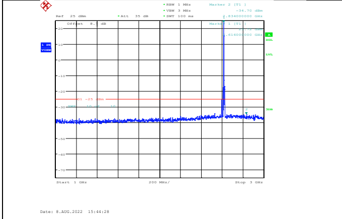
Band38-5MHz-QPSK-38225-1RB#0-Range2:1000~3000MHz
