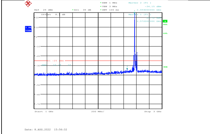
Band38-20MHz-16QAM-37850-1RB#0-Range2:1000~3000MHz
