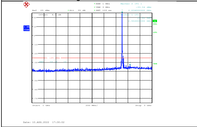
Band7-5MHz-QPSK-20775-1RB#0- Range2:1000~3000MHz
