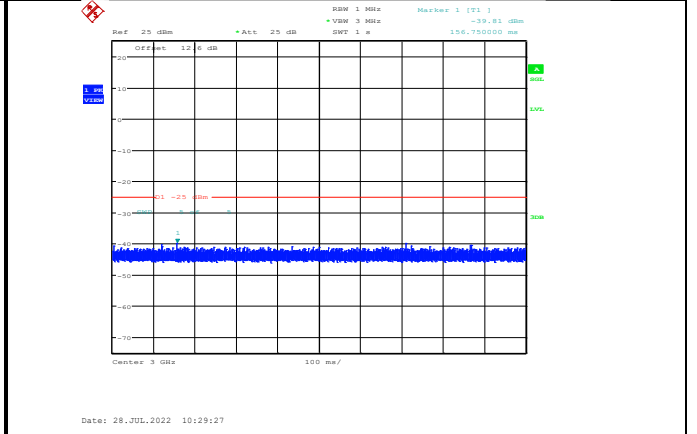
Band7-10MHz-QPSK-20800-1RB#0-Range3:3000~27000MHz
