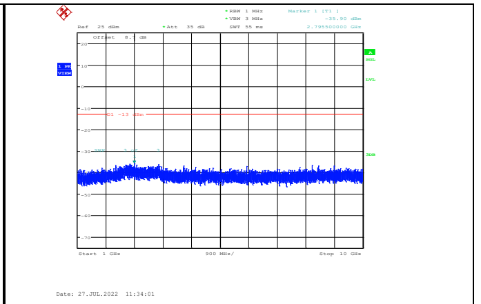
Band5-10MHz-QPSK-20525-1RB#0- Range2:1000~10000MHz
