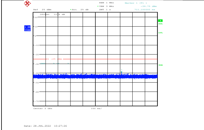
Band7-5MHz-QPSK-21425-1RB#0-Range3:3000~27000MHz
