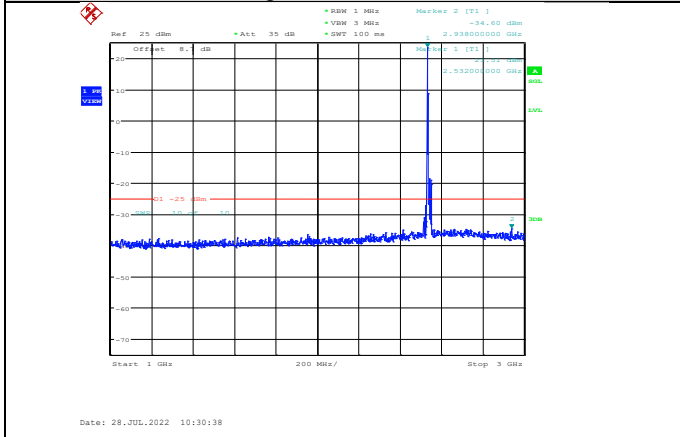
Band7-10MHz-QPSK-21100-1RB#0-Range2:1000~3000MHz
