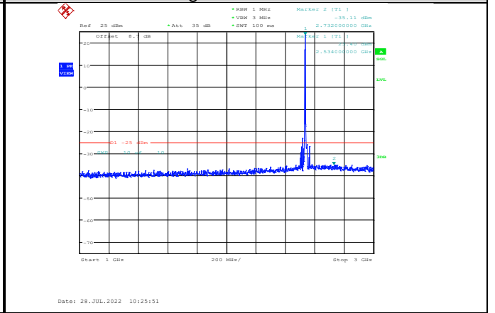
Band7-5MHz-QPSK-21100-1RB#0- Range2:1000~3000MHz
