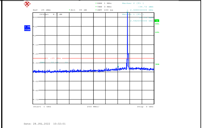
Band7-10MHz-QPSK-21400-1RB#0-Range2:1000~3000MHz
