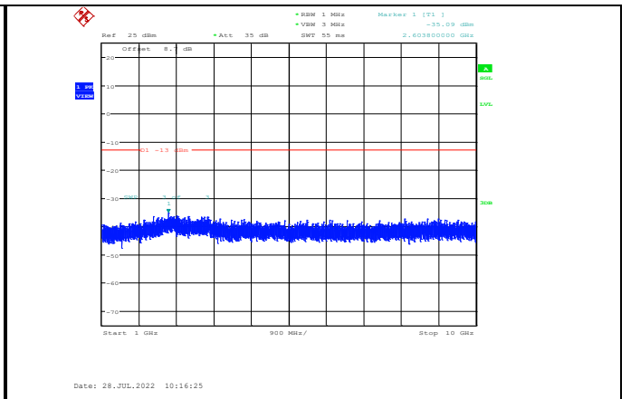
Band5-5MHz-QPSK-20525-1RB#0- Range2:1000~10000MHz
