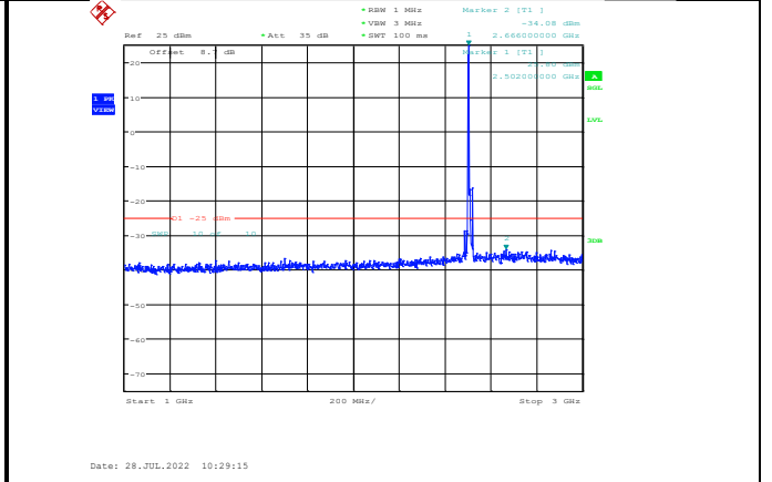
Band7-10MHz-QPSK-20800-1RB#0-Range2:1000~3000MHz
