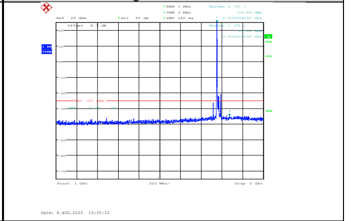
Band7-20MHz-QPSK-21350-1RB#0-Range2:1000~3000MHz
