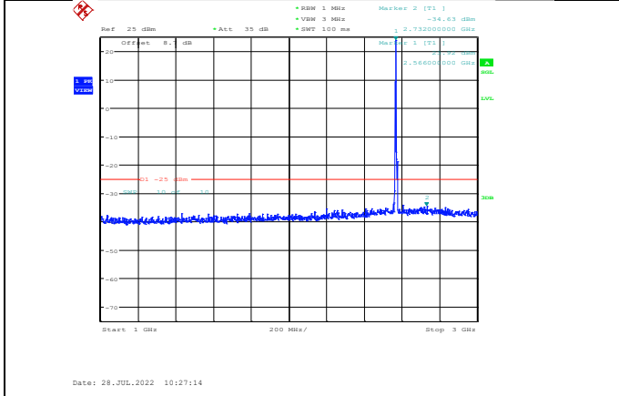
Band7-5MHz-QPSK-21425-1RB#0-Range2:1000~3000MHz
