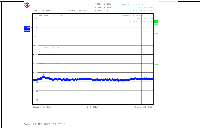
EGPRS1900-661-2-1000~20000MHz
