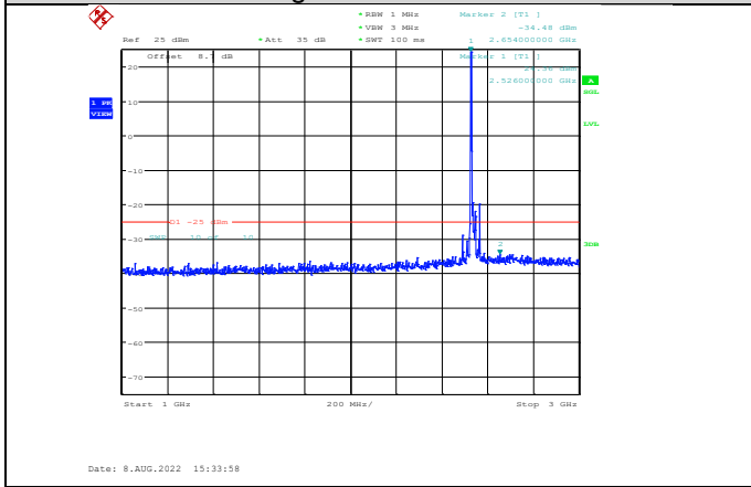
Band7-20MHz-QPSK-21100-1RB#0-Range2:1000~3000MHz
