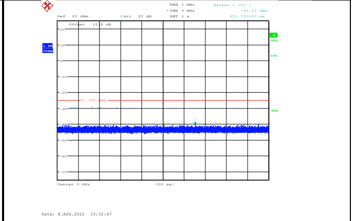
Band7-20MHz-QPSK-20850-1RB#0-Range3:3000~27000MHz
