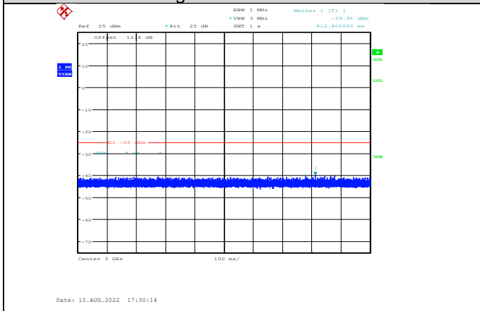
Band7-5MHz-QPSK-20775-1RB#0- Range3:3000~27000MHz
