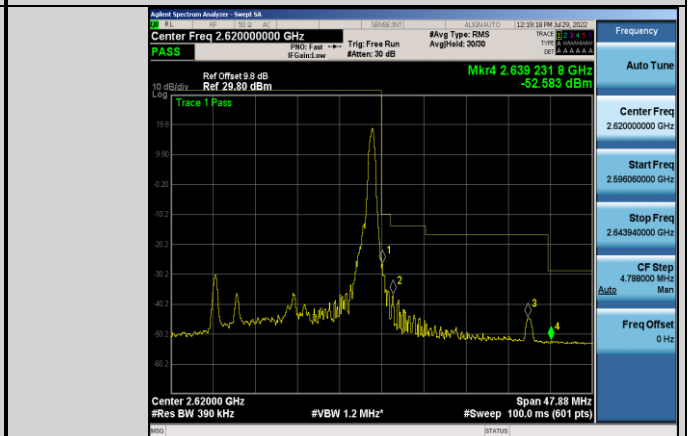
Band38-20MHz-QPSK-38150-1RB#99
