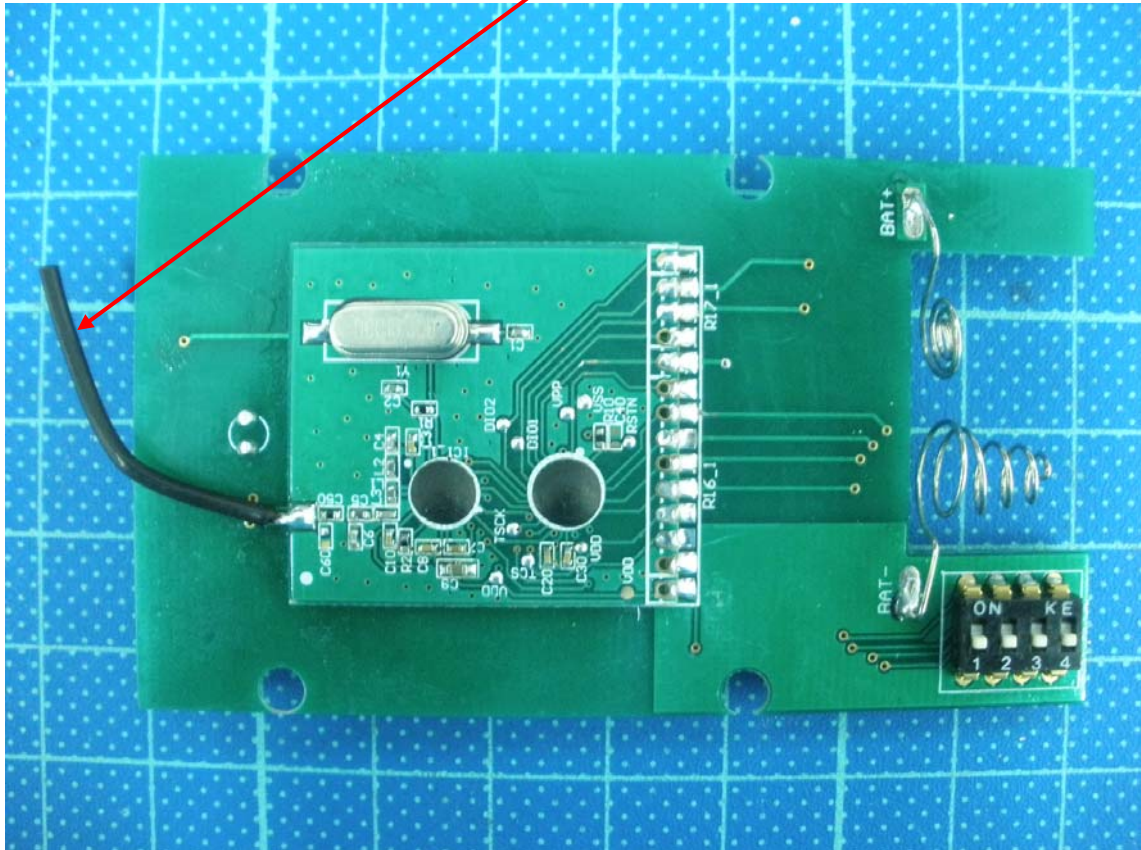
Antenna
