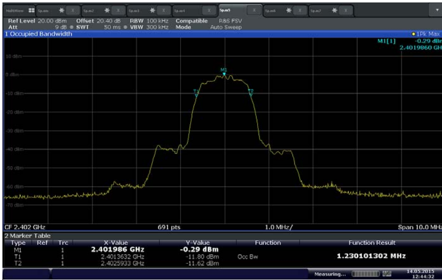
\pi/4 -DQPSK Low Channel
