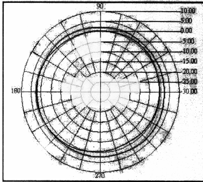
H-plane For 2.4 GHz
