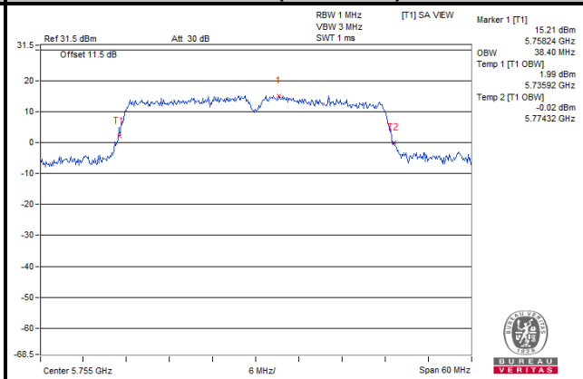
Ch 151 (5755 MHz)
