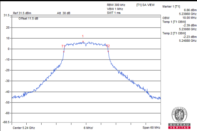
Ch 48 (5240 MHz)
