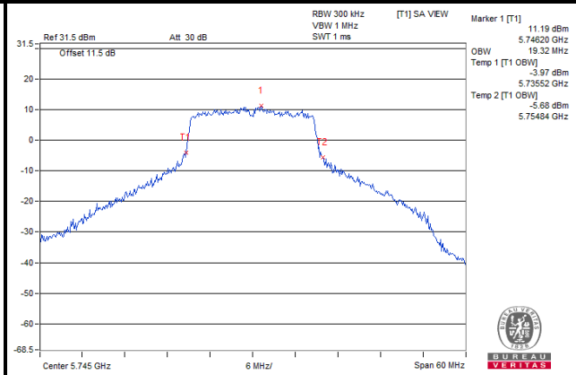
Ch 149 (5745 MHz)
