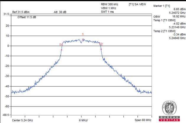
Ch 48 (5240 MHz)
