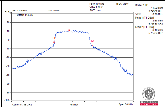
Ch 149 (5745 MHz)
