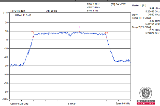
Ch 46 (5230 MHz)
