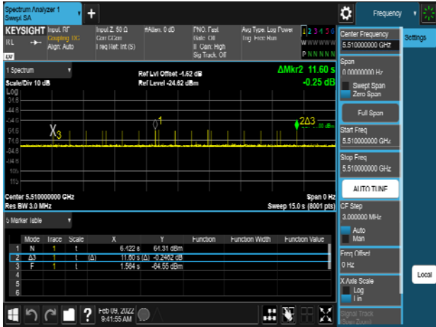
HT40_5510MHz_Radar_Type 6
