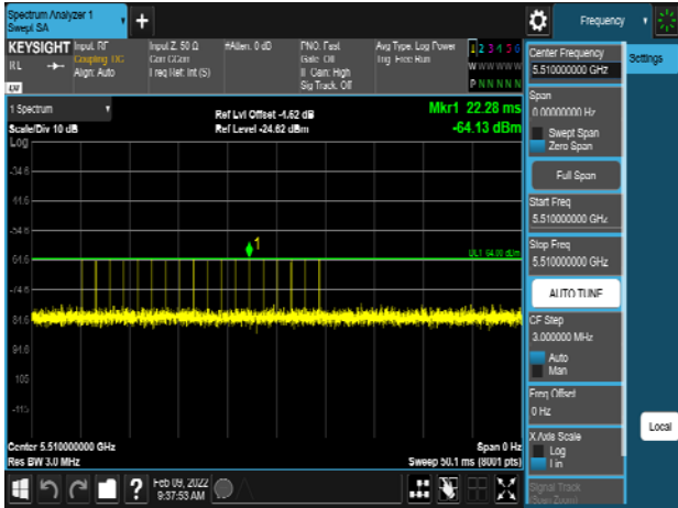
HT40_5510MHz_Radar_Type 1-A
