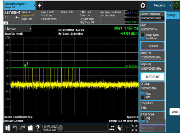
VHT80_5530MHz_Radar_Type 5
