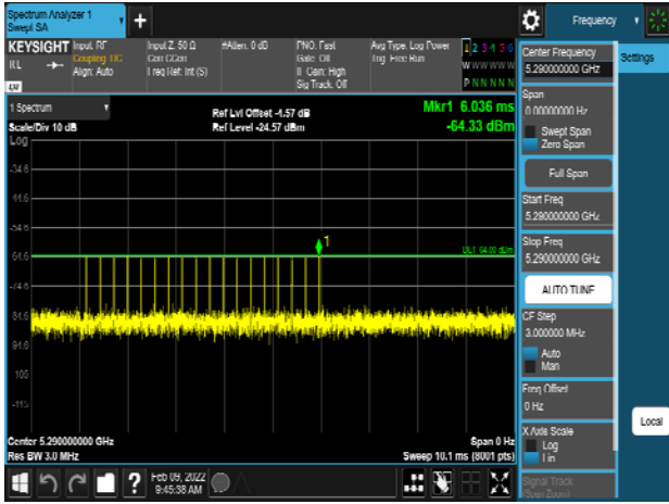
VHT80_5290MHz_Radar_Type 4
