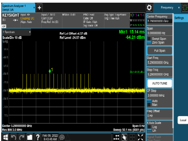
VHT80_5290MHz_Radar_Type 0
