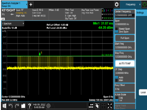
VHT80_5530MHz_Radar_Type 2
