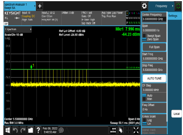
VHT80_5530MHz_Radar_Type 1-A
