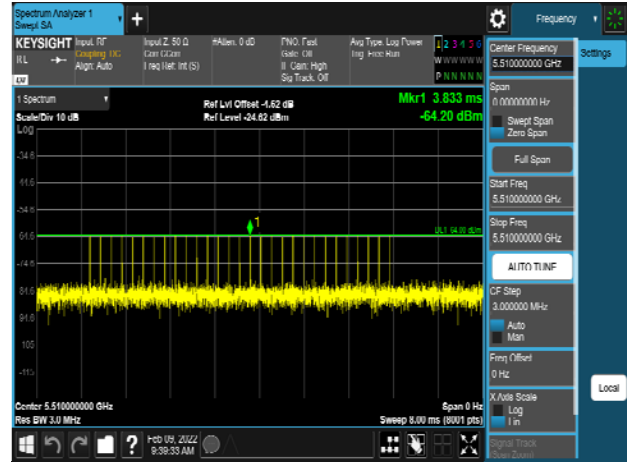
HT40_5510MHz_Radar_Type 3
