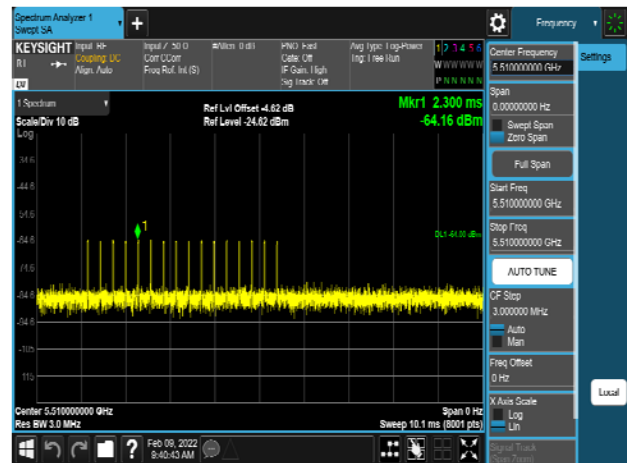
HT40_5510MHz_Radar_Type 4
