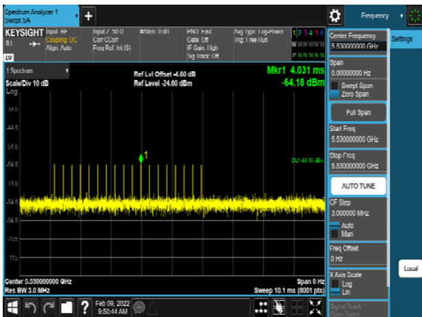
VHT80_5530MHz_Radar_Type 3
