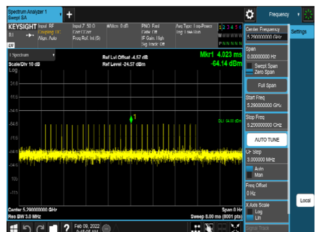
VHT80_5290MHz_Radar_Type 2
