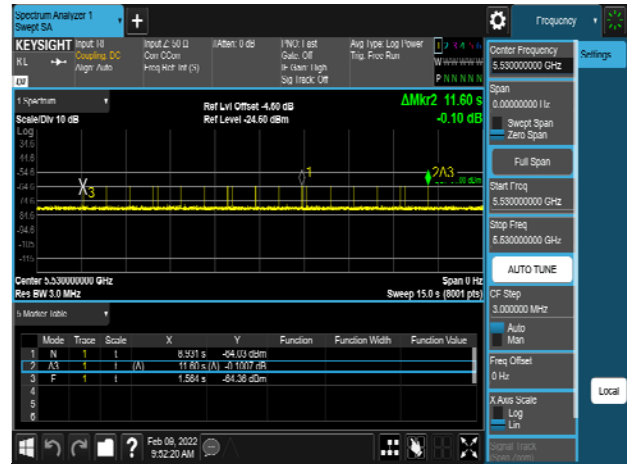
VHT80_5530MHz_Radar_Type 6
