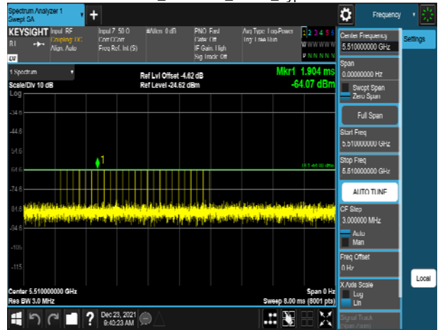
HT40_5510MHz_Radar_Type 3
