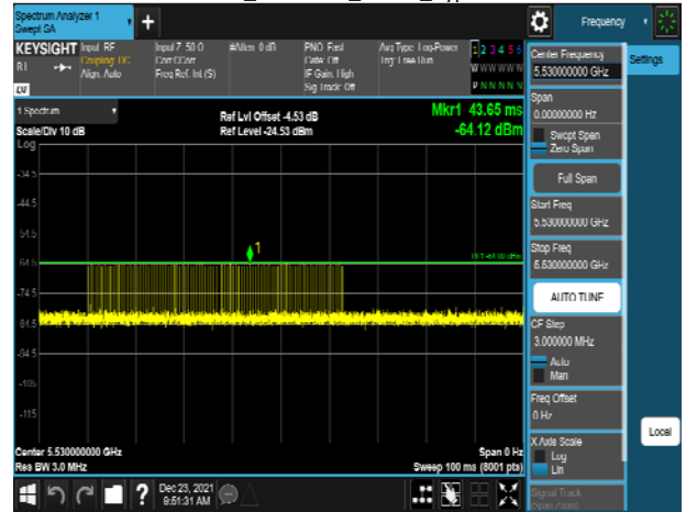
VHT80_5530MHz_Radar_Type 1-A
