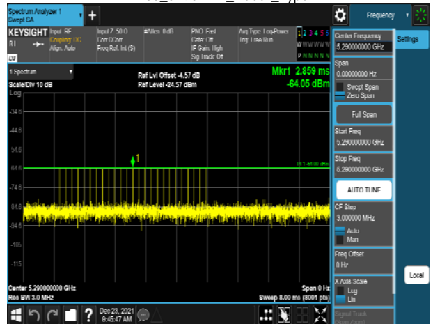
VHT80_5290MHz_Radar_Type 2
