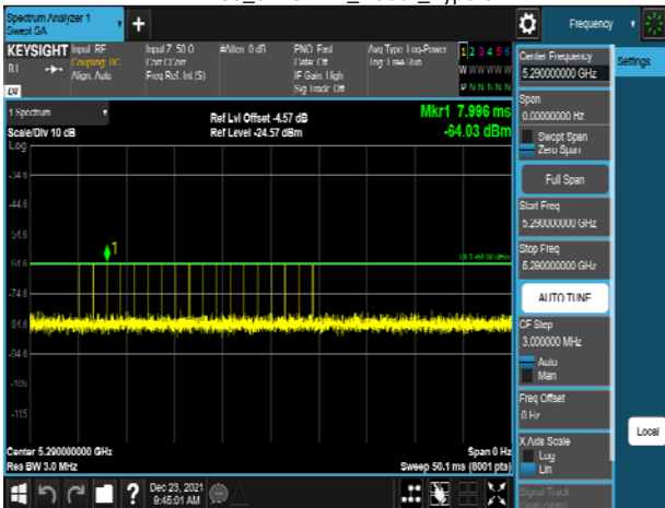
VHT80_5290MHz_Radar_Type 0
