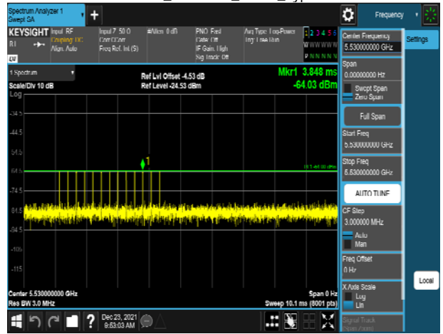
VHT80_5530MHz_Radar_Type 5
