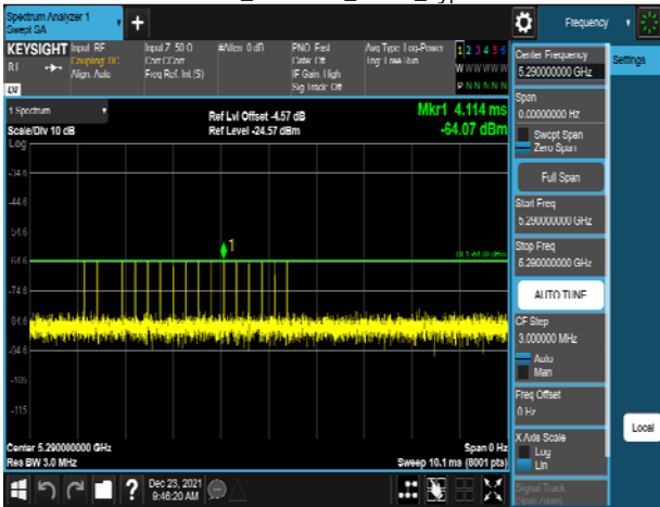
VHT80_5290MHz_Radar_Type 4
