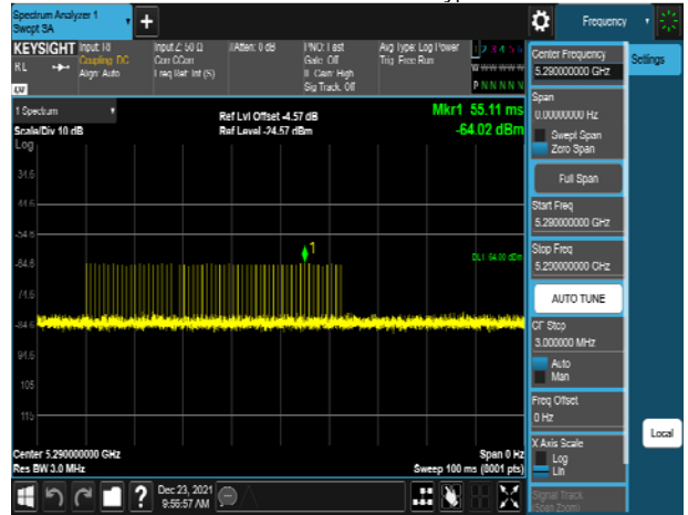
VHT80_5290MHz_Radar_Type 2
