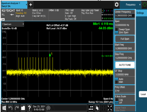
VHT80_5290MHz_Radar_Type 5
