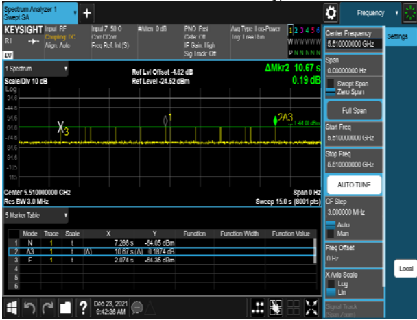
HT40_5510MHz_Radar_Type 6
