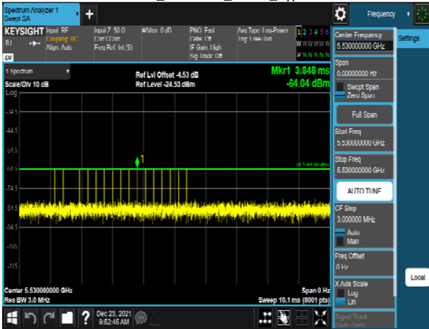
VHT80_5530MHz_Radar_Type 3
