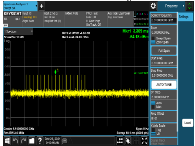
HT40_5510MHz_Radar_Type 4
