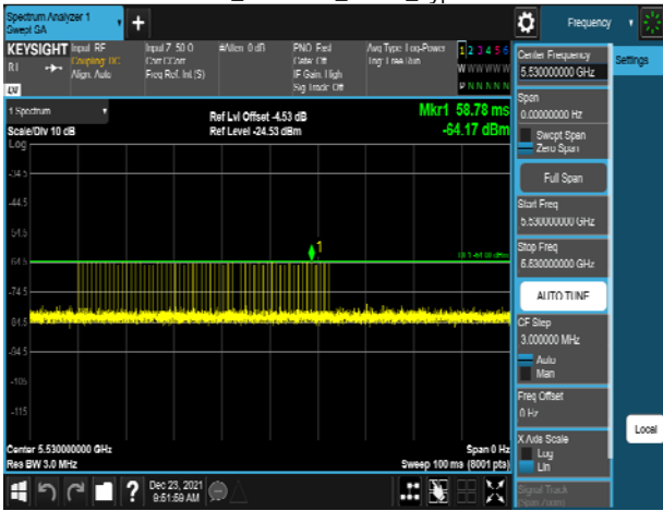
VHT80_5530MHz_Radar_Type 2
