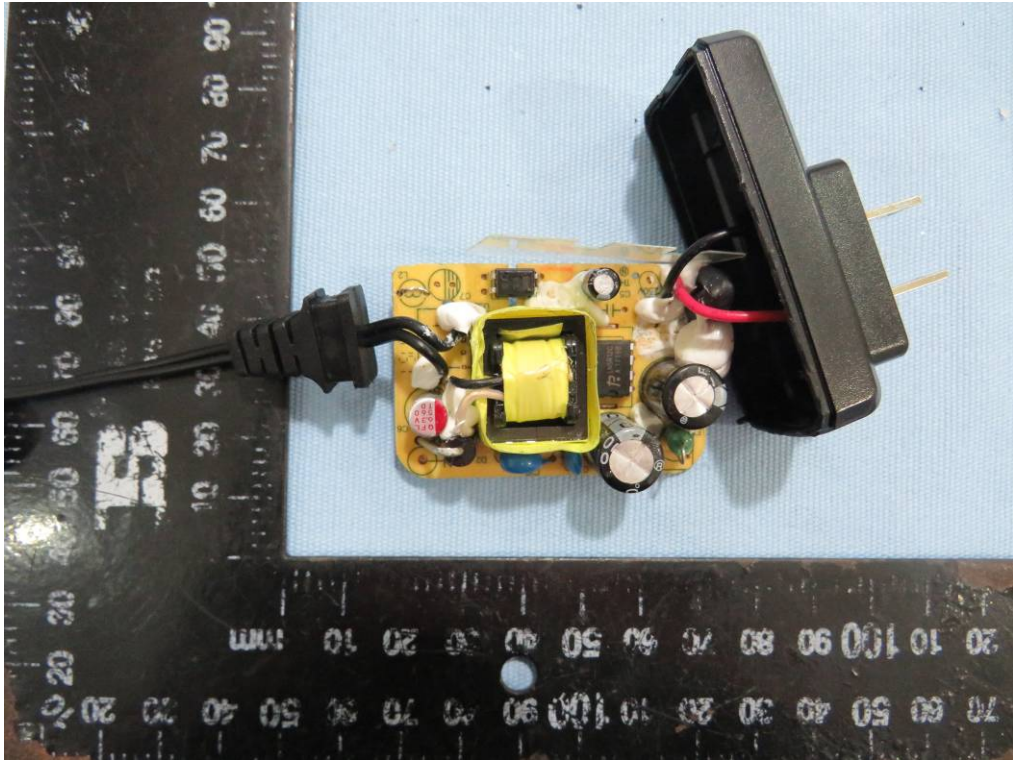
Adapter: ZAU-A050120A-04
