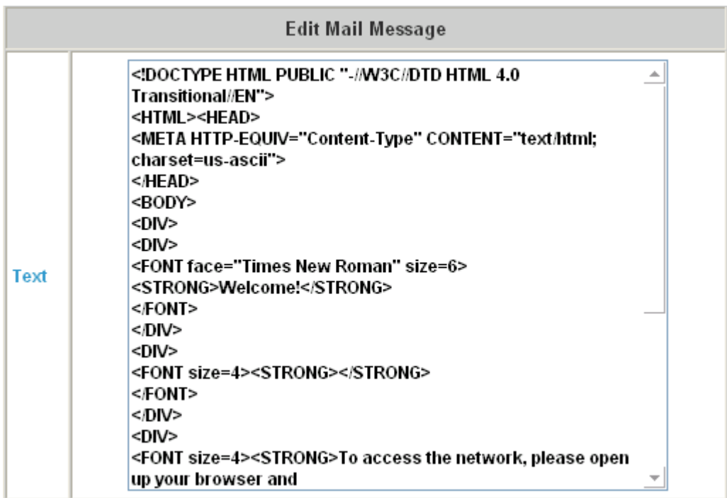
Figure 5-75 POP3 Message
