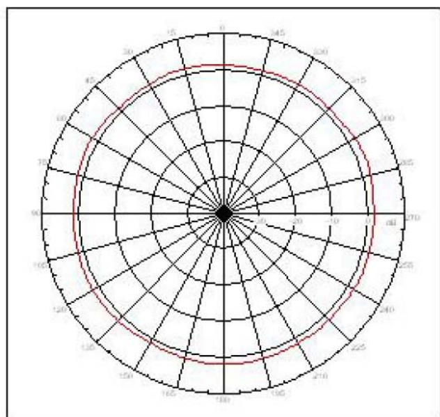
2.45GHz_H-plane
