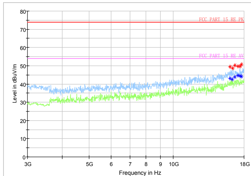
BT_DH5_CH78
