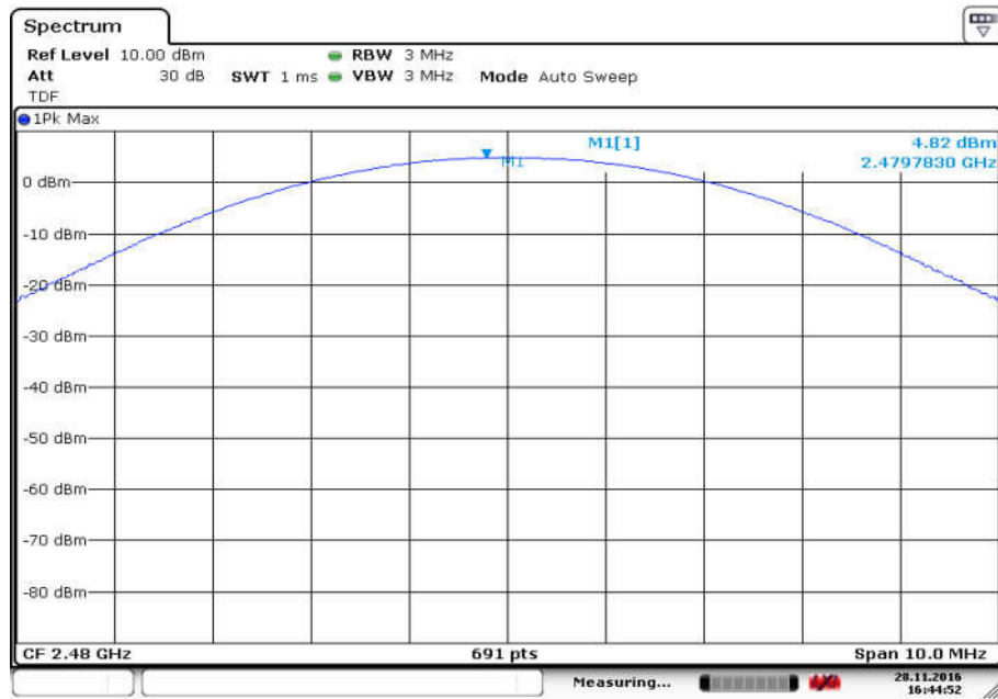
Fig. 5 Maximum Peak Output Power( \pi/4 DQPSK, Ch 39)
