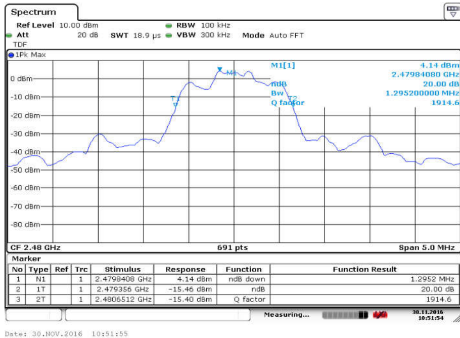
Fig. 88 Occupied 20dB Bandwidth ( \pi/4 DQPSK, Ch 78)
