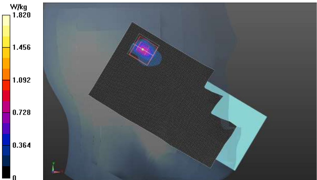
Fig.41 WLAN 5G
