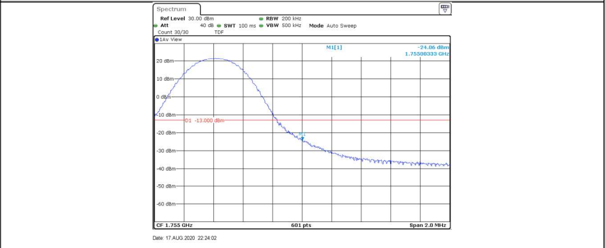
Band4-10MHz-QPSK-20350-1RB#0
