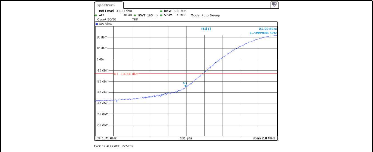
Band4-20MHz-QPSK-20050-100RB#0
