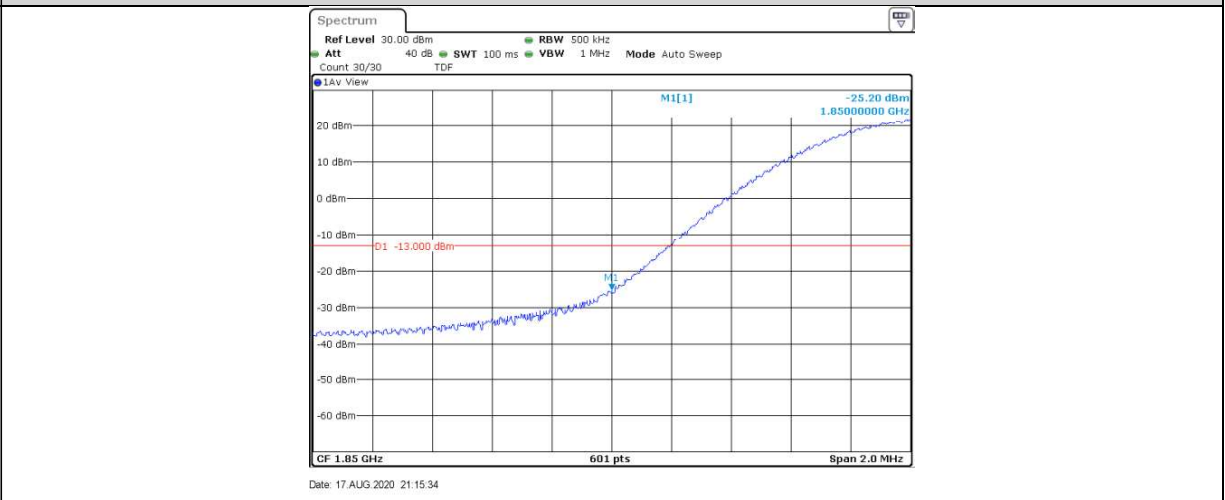
Band2-20MHz-16QAM-18700-1RB#99
