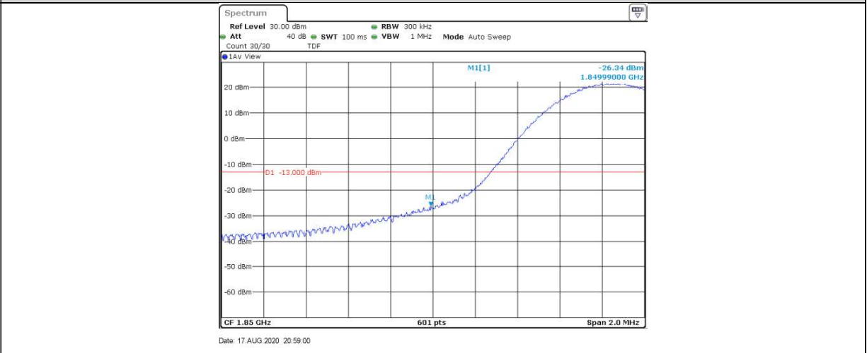
Band2-15MHz-16QAM-18675-1RB#74
