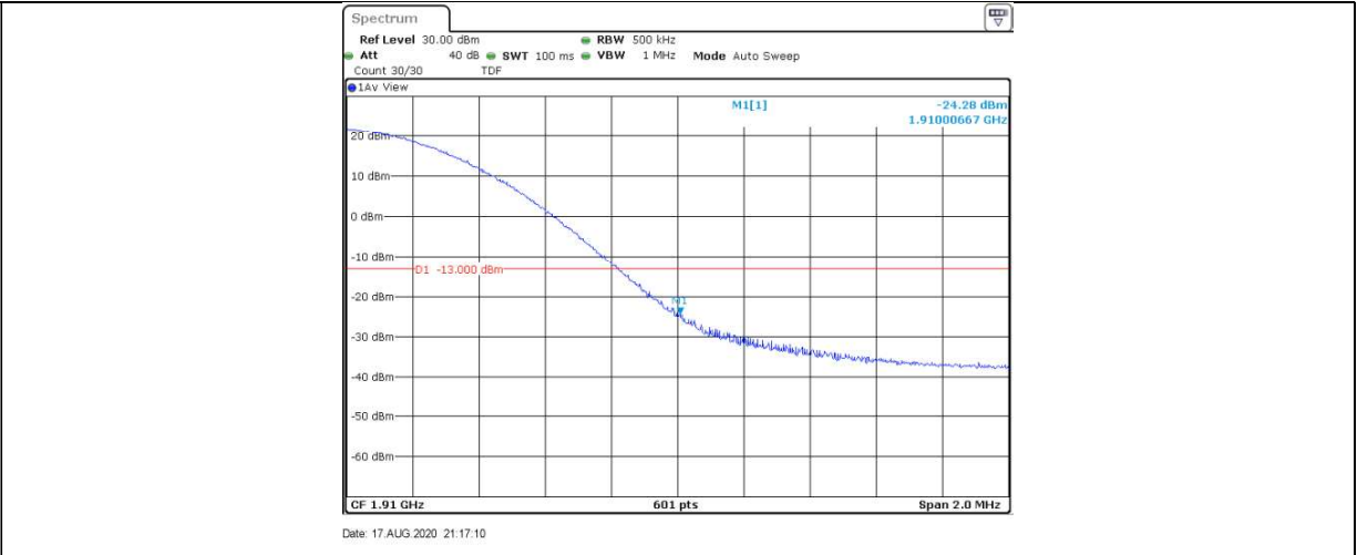
Band2-20MHz-QPSK-19100-100RB#0
