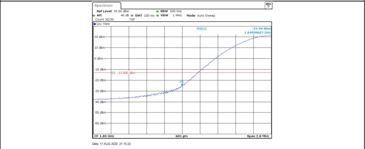
Band2-20MHz-QPSK-18700-1RB#99
