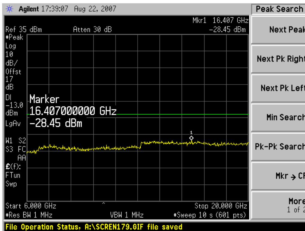
Channel 661, 6GHz~20GHz
