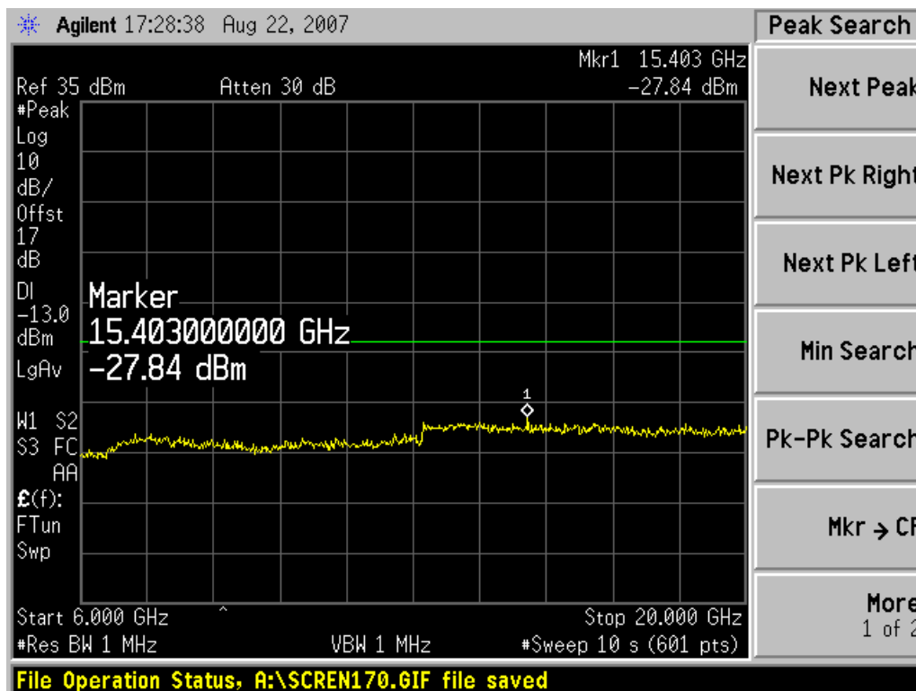
Channel 661, 6GHz~20GHz
