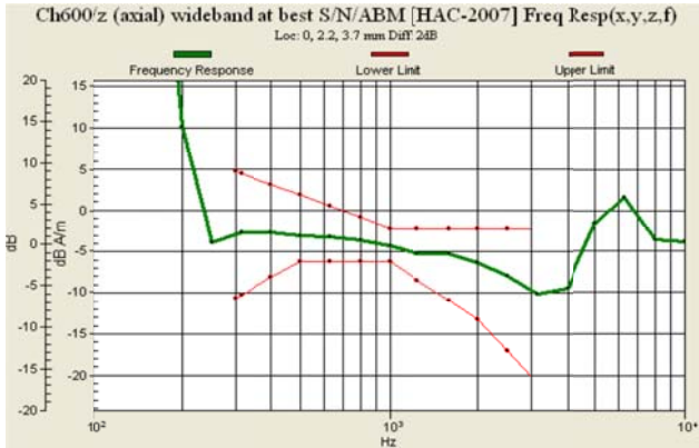
Fig. 9.5 CDMA2000 BC1 Ch600
