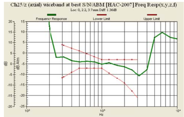
Fig. 9.4 CDMA2000 BC1 Ch25
