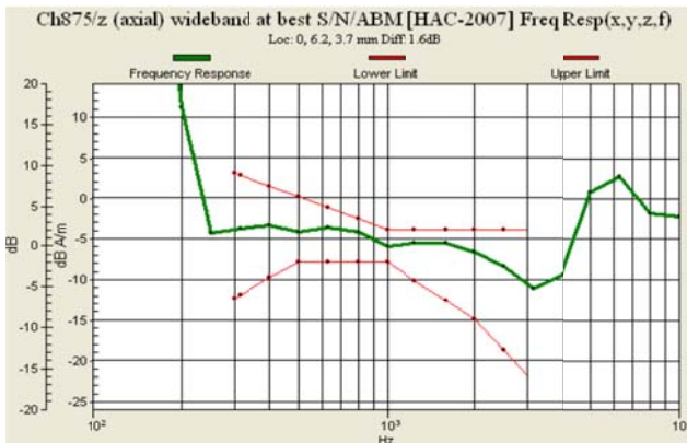
Fig. 9.9 CDMA2000 BC15 Ch875
