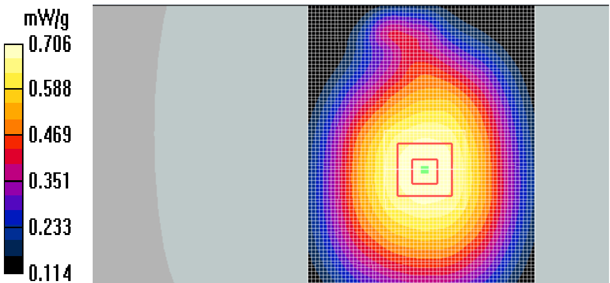
Fig.6 WCDMA 850 CH4182
