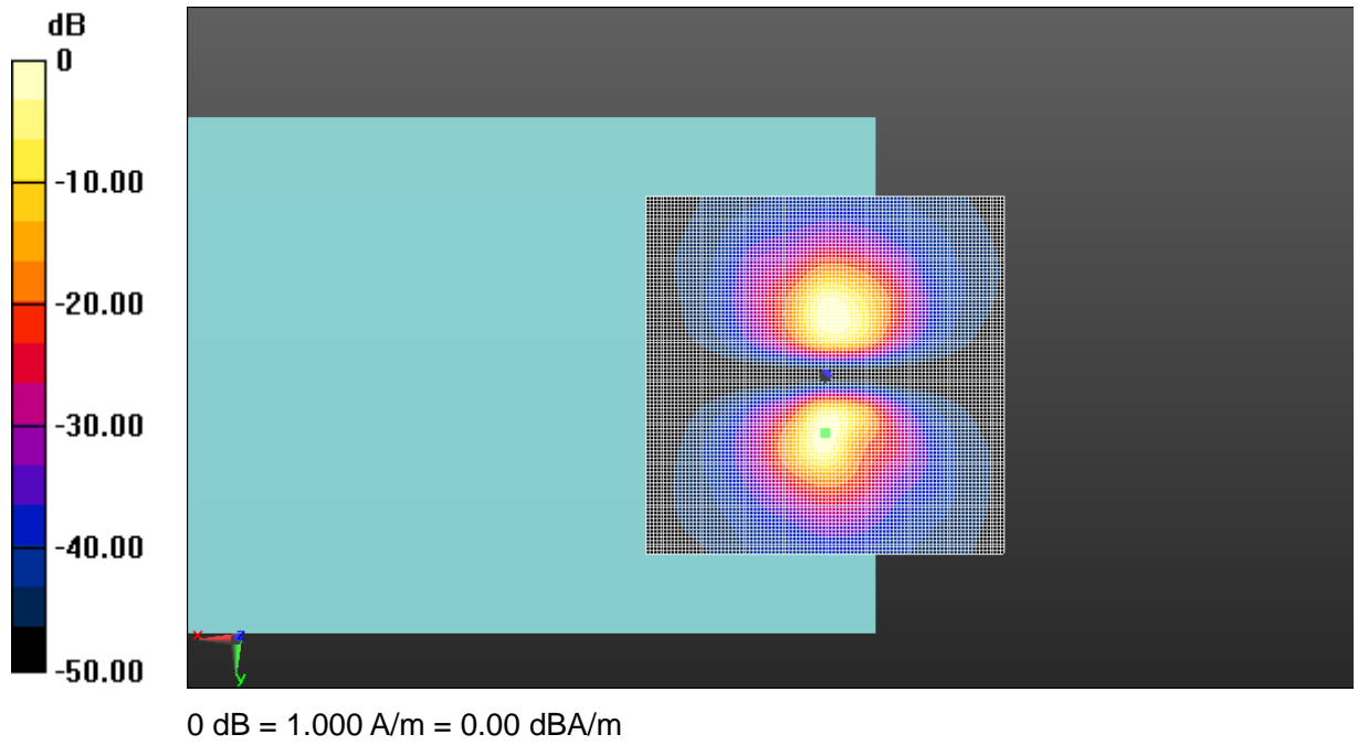
Fig A.6 T-Coil CDMA BC0
