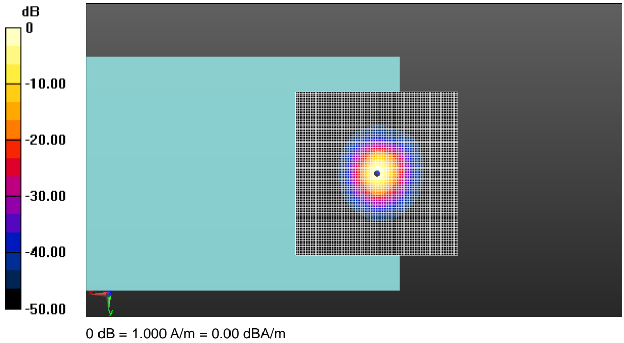
Fig A.5 T-Coil CDMA BC0
