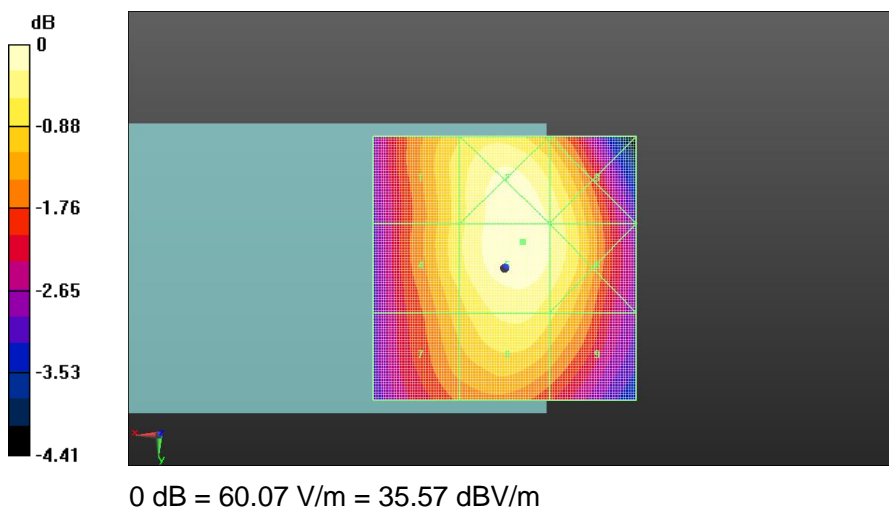
Fig A.3 HAC RF E-Field GSM 850 Low
