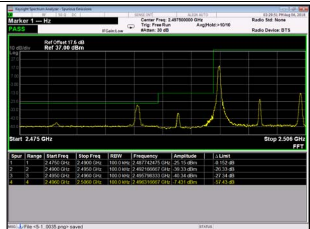
LowRange_TDD41_10MHz_2501_OneRB_low_Q16
