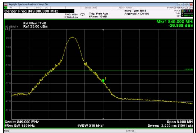
HighRange_FDD26_15MHz_841.5_fullIRB_HighQ16
