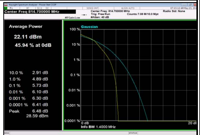
FDD26_1.4MHz_814.7MHz_fullIRB_Q16
