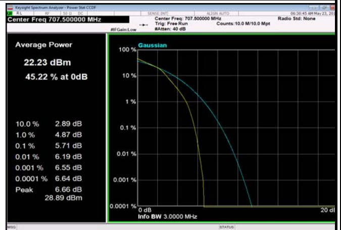
FDD12_5MHz_707.5MHz_fullRB_Q16
