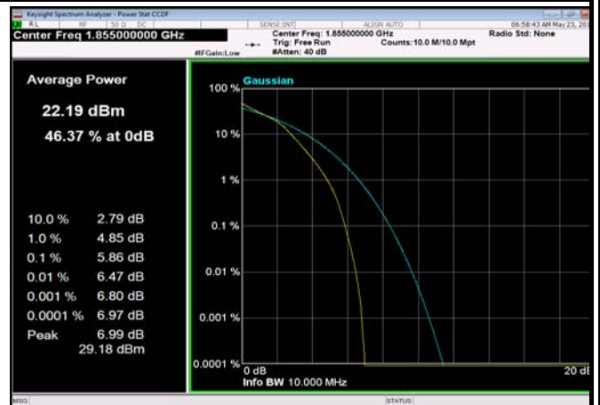
FDD25_10MHz_1855MHz_fullRB_Q16
