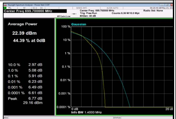
FDD12_1.4MHz_699.7MHz_fullRB_Q16
