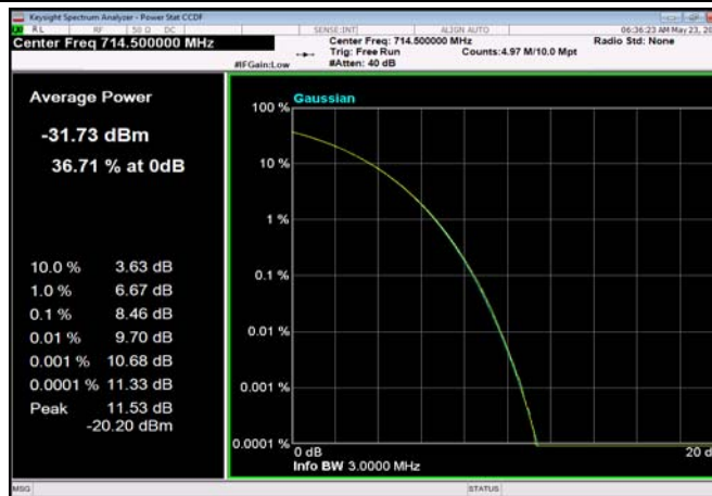
FDD12_3MHz_714.5MHz_OneRB_high_Q16
