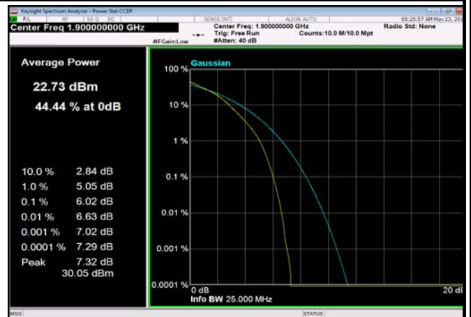
FDD02_20MHz_1900MHz_fullRB_Q16
