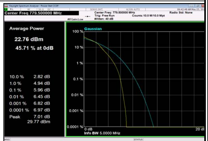
FDD13_5MHz_779.5MHz_fullRB_Q16
