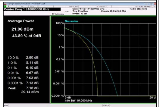
FDD25_10MHz_1910MHz_fullRB_Q16
