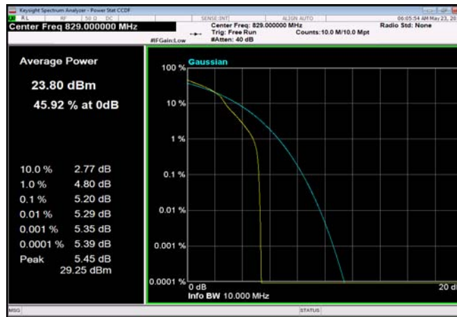
FDD05_10MHz_829MHz_OneRB_high_Q16
