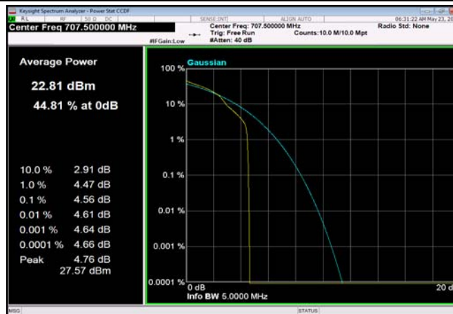
FDD12_5MHz_707.5MHz_OneRB_high_Q16
