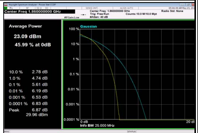
FDD02_20MHz_1860MHz_fullRB_Q16
