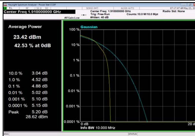
FDD25_10MHz_1910MHz_OneRB_high_Q16
