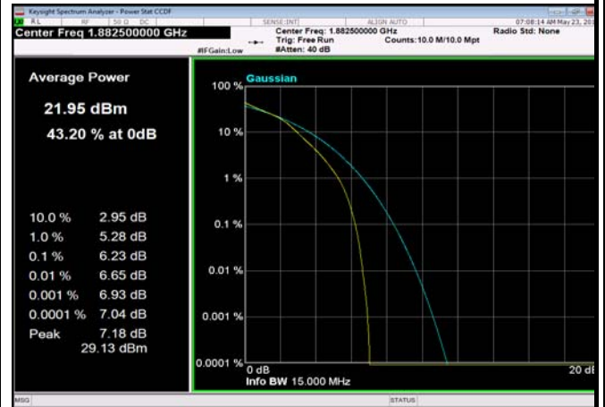
FDD25_20MHz_1882.5MHz_fullIRB_Q16
