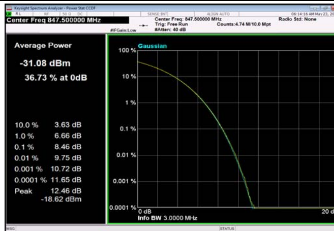
FDD05_3MHz_847.5MHz_OneRB_high_Q16
