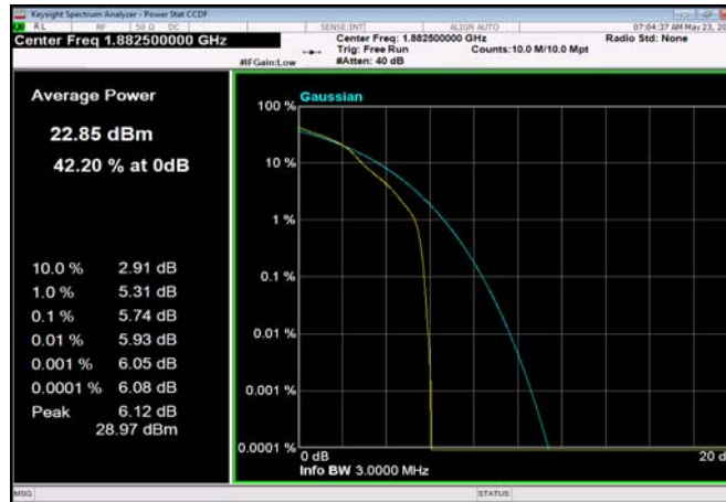
FDD25_5MHz_1882.5MHz_OneRB_high_Q16
