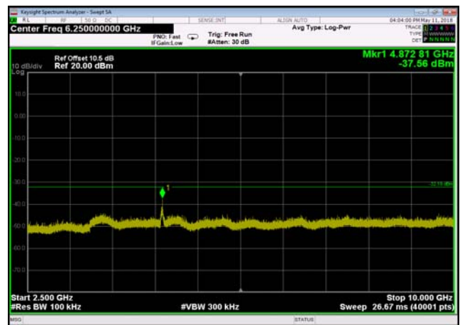
802.11n(HT40),2437MHz,Ant0,Plot 4,2500MHz~10000MHz
