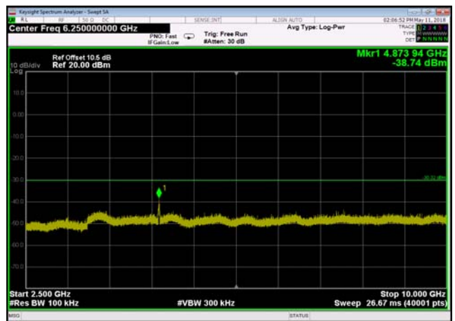
802.11g,2437MHz,Ant0,Plot 4,2500MHz~10000MHz
