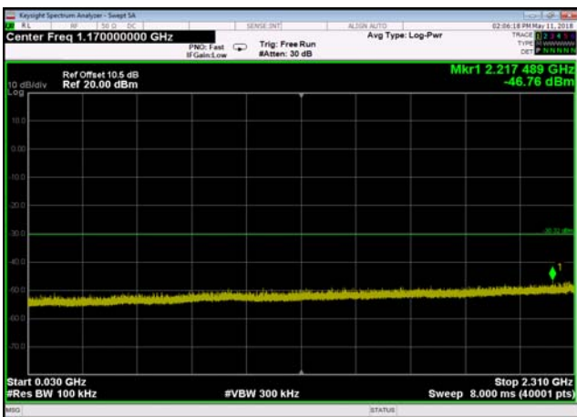
802.11g,2437MHz,Ant0,Plot 3,30MHz~2310MHz
