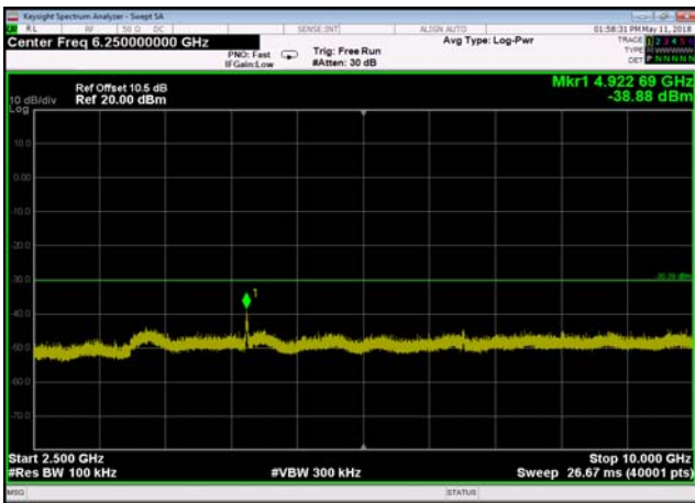
802.11g,2462MHz,Ant0,Plot 4,2500MHz~10000MHz
