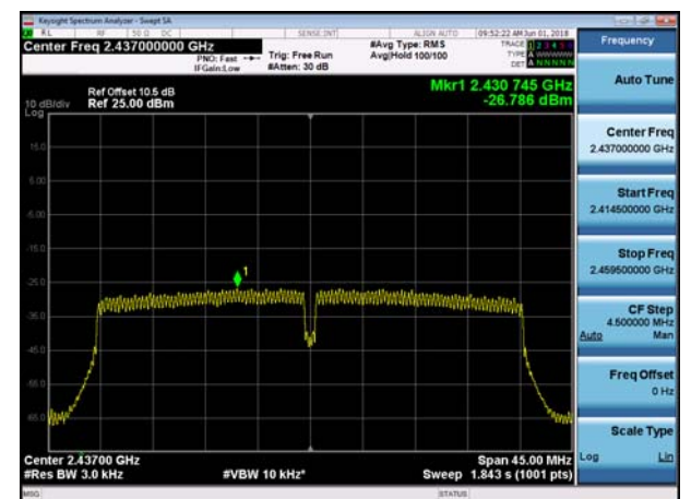
802.11n(HT40),2437MHz,Ant0
