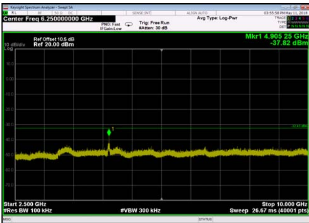
802.11n(HT40),2452MHz,Ant0,Plot 4,2500MHz~10000MHz
