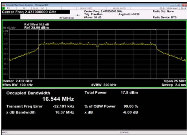
802.11g,2437MHz,Ant0
