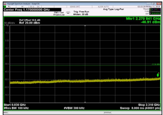
802.11n(HT40),2422MHz,Ant0,Plot 3,30MHz~2310MHz
