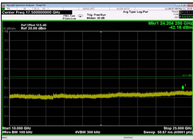
802.11b,2412MHz,Ant0,Plot 5,10000MHz~25000MHz
