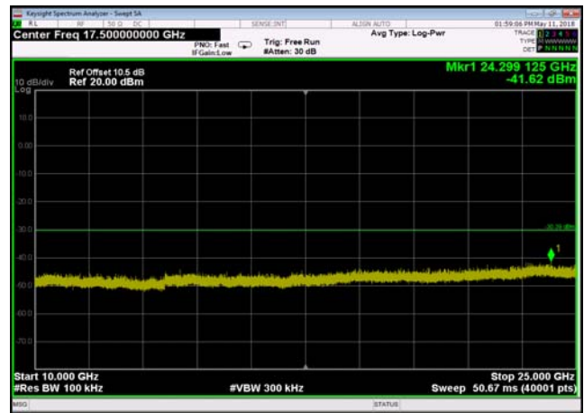
802.11g,2462MHz,Ant0,Plot 5,10000MHz~25000MHz
