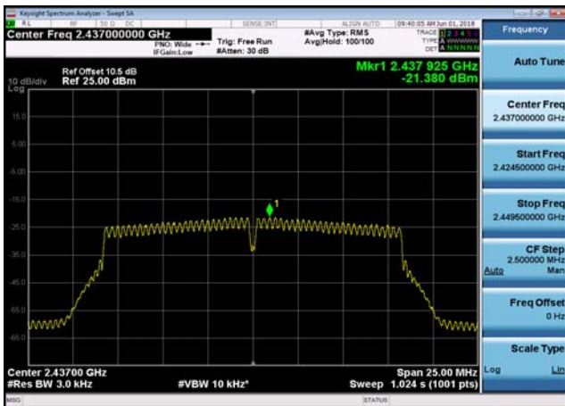
802.11g,2437MHz,Ant0
