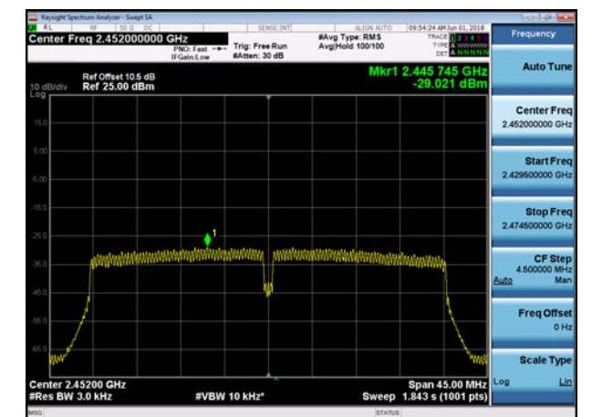
802.11n(HT40),2452MHz,Ant0
