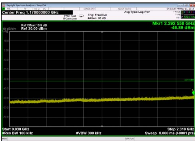
802.11n(HT40),2437MHz,Ant0,Plot 3,30MHz~2310MHz
