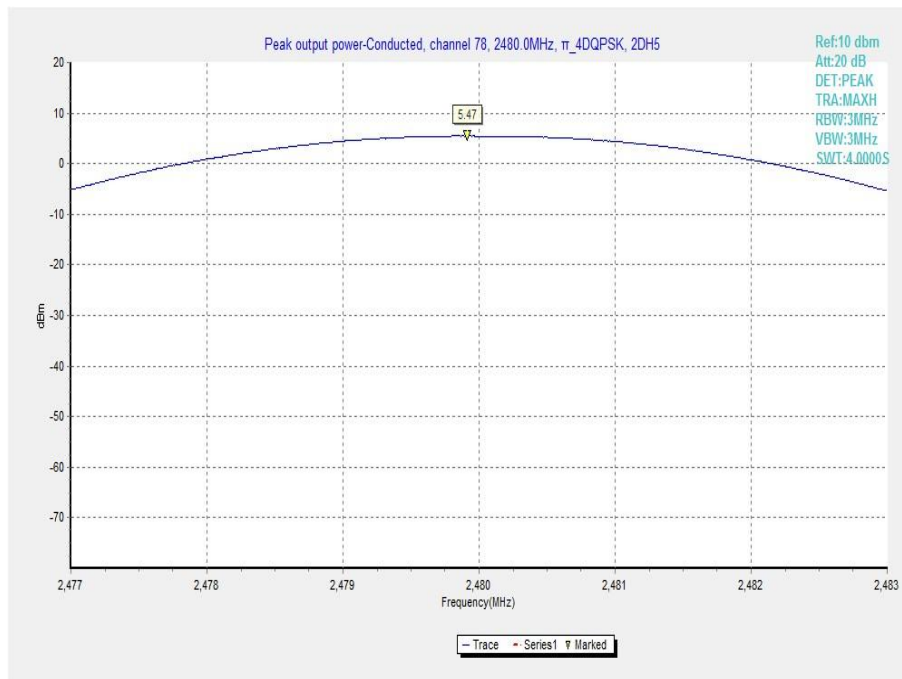
Fig. 6 Maximum Peak Output Power( \pi /4 DQPSK, Ch 78)
