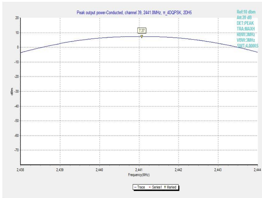
Fig. 5 Maximum Peak Output Power( \pi /4 DQPSK, Ch 39)
