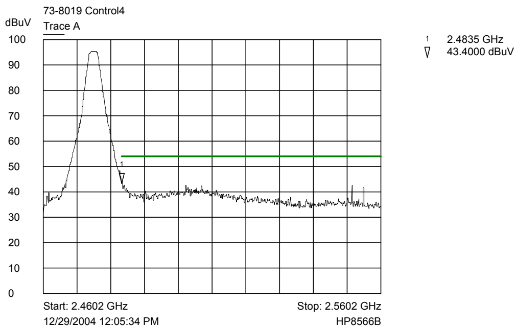
Trace A Upper Band Edge
