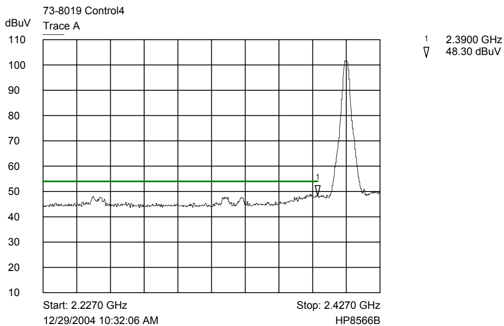
Trace A Lower Band Edge
