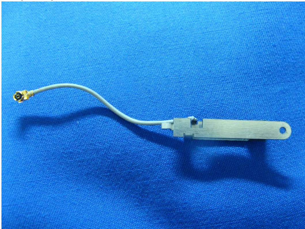
(10) EUT Photo (Antenna)
