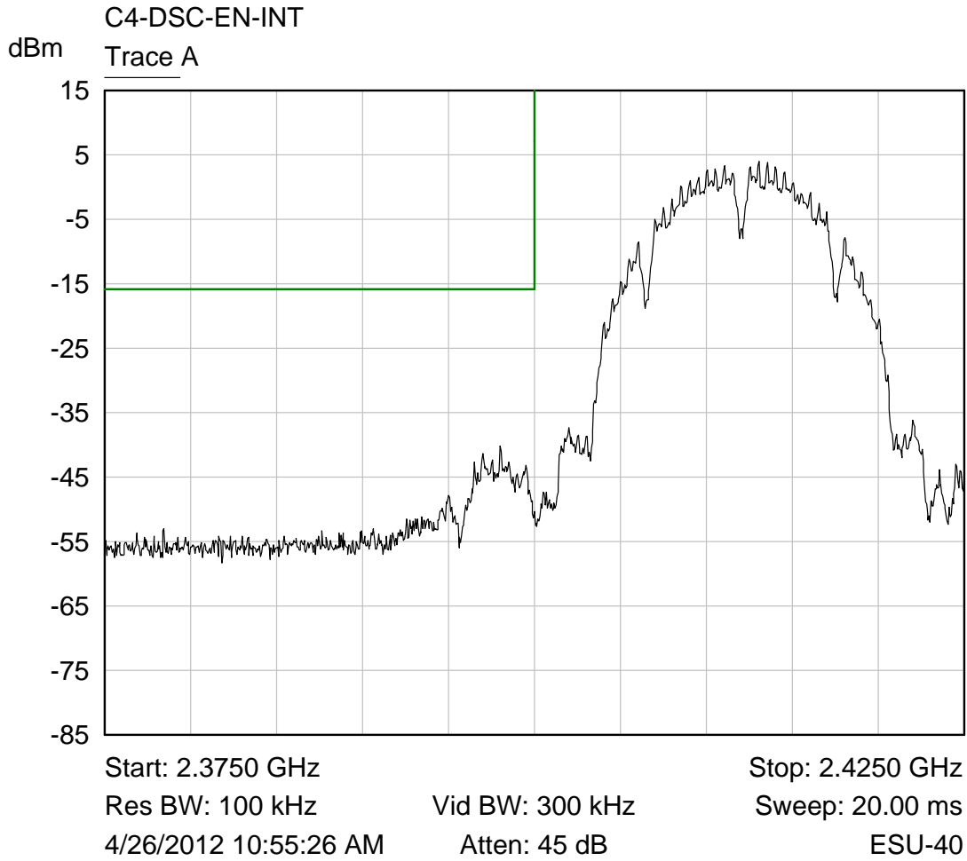
Trace A Band edge
