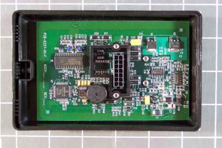
XF1560CS2 - Enclosure
