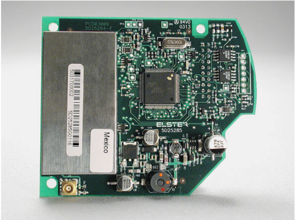
LAN Board
