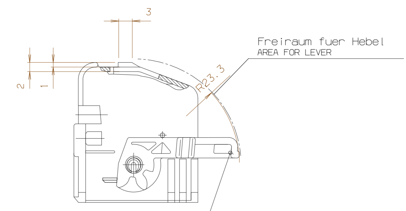
Untersicht (ohne Kabel)
