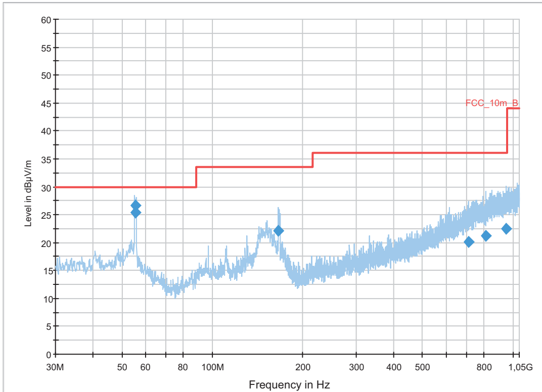
FCC_10m(B)_3
