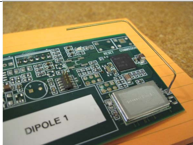
Wire dipole: Bend 1
