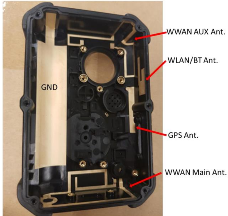
WLAN Ant.
