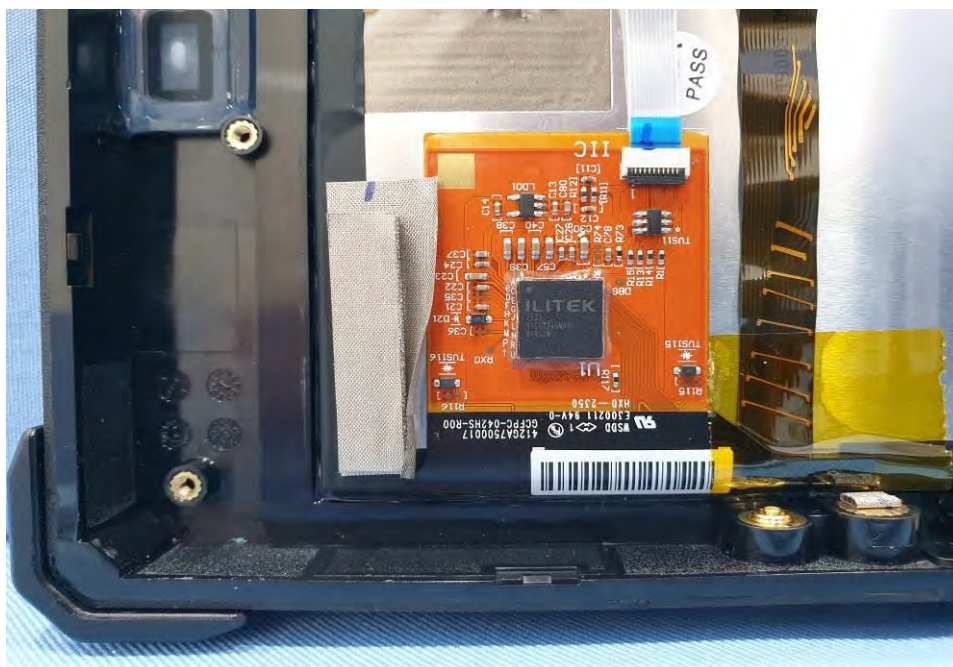
EUT Photo (94)
