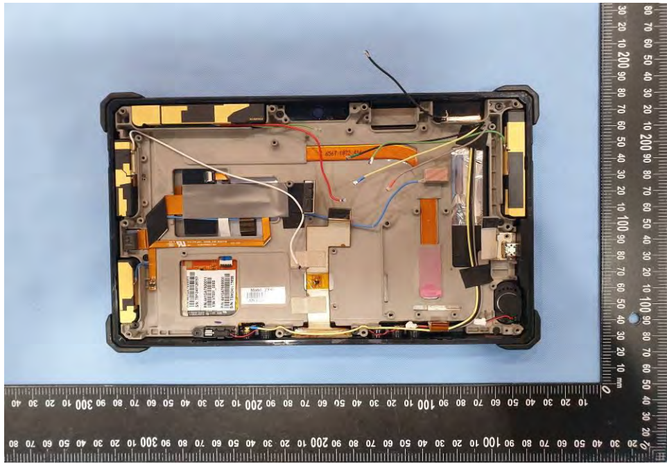
EUT Photo (62)
