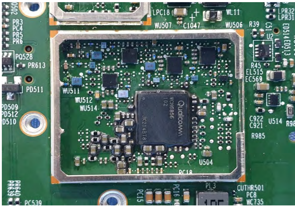
EUT Photo (50)
