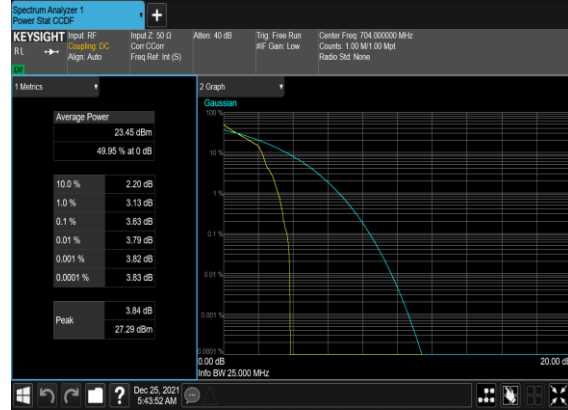
B2_N12(10M)_DFT-s-OFDM_PI_2-BPSK_Edge_1RB_Left_Low_CH
