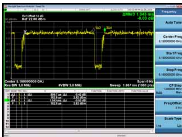
802.11n(40MHz)
