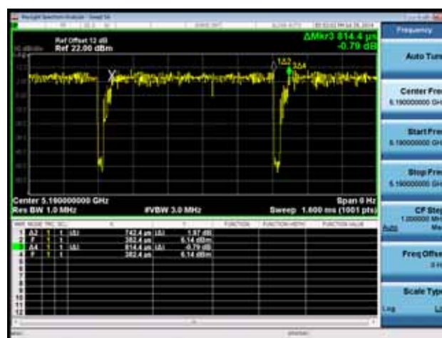
802.11ax(40MHz)
