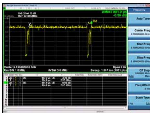
802.11ac(40MHz)
