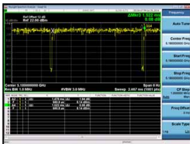
802.11ax(20MHz)
