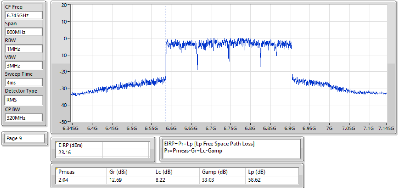
EIRP;Band:6.7G;be320;BWch:320MHz;Nss:1,(M0);Nant:2;Ch:6745MHz;TX
