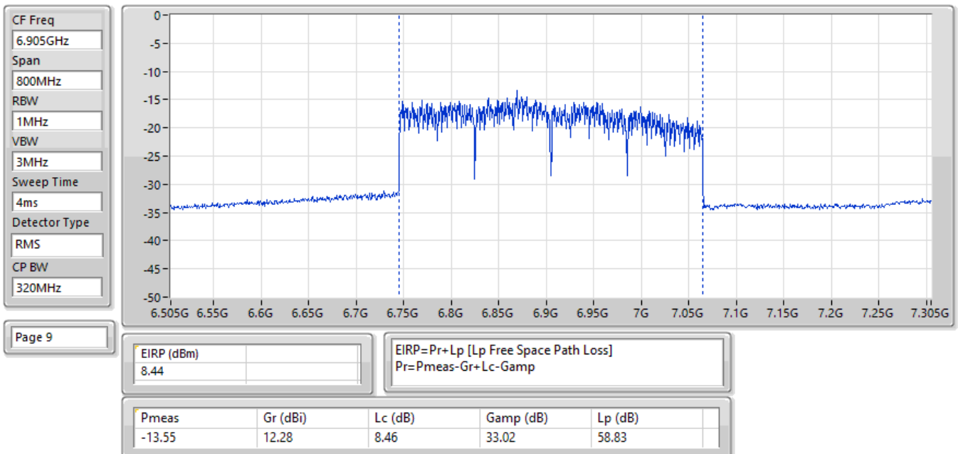
EIRP;Band:6.7G;be320;BWch:320MHz;Nss:1,(M0);Nant:2;Ch:6905MHz;TX
