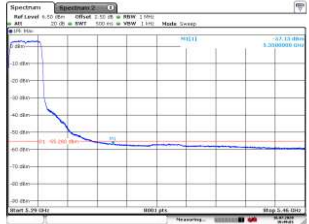
5300MHz with 2*2 Beamforming AV
