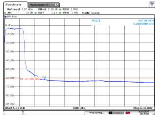
5320MHz with 4*4 Beamforming AV
