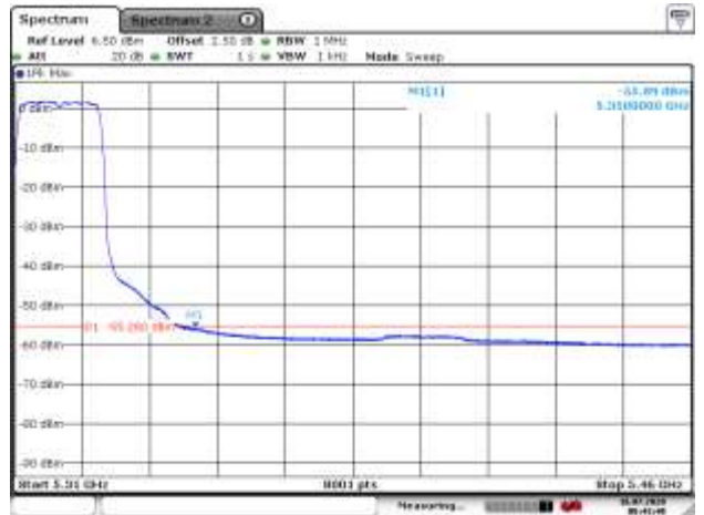
5320MHz with 2*2 CDD AV
