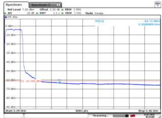
5300MHz with 4*4 Beamforming AV
