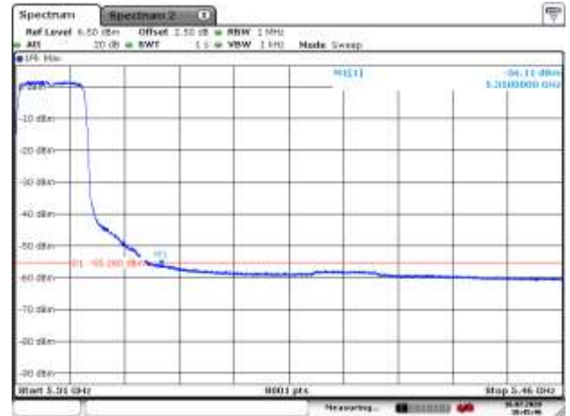
5320MHz with 2*2 Beamforming AV
