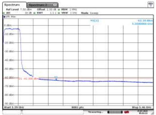
5300MHz with 4*4 CDD AV
