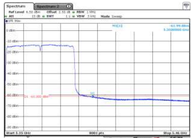
5290MHz with 4*4 Beamforming AV
