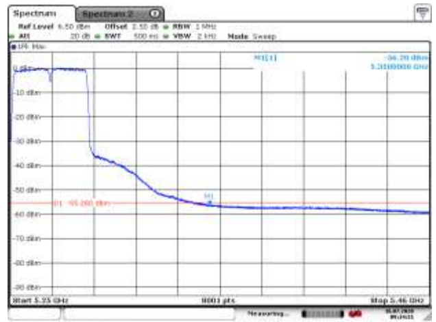
5270MHz with 2*2 CDD AV
