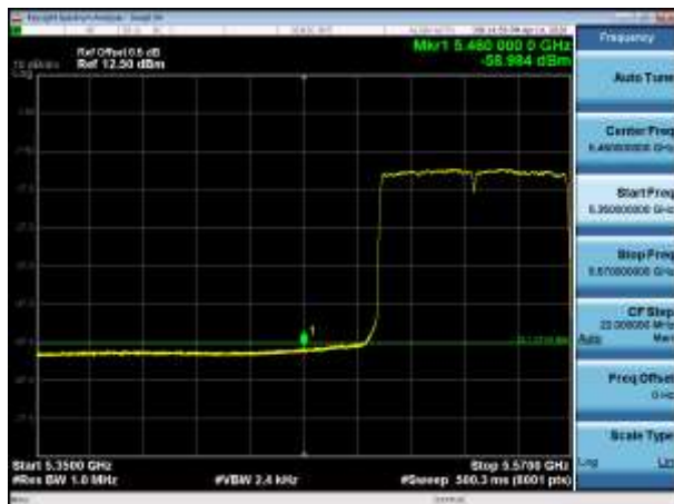
5530MHz with 4*4 Beamforming AV
