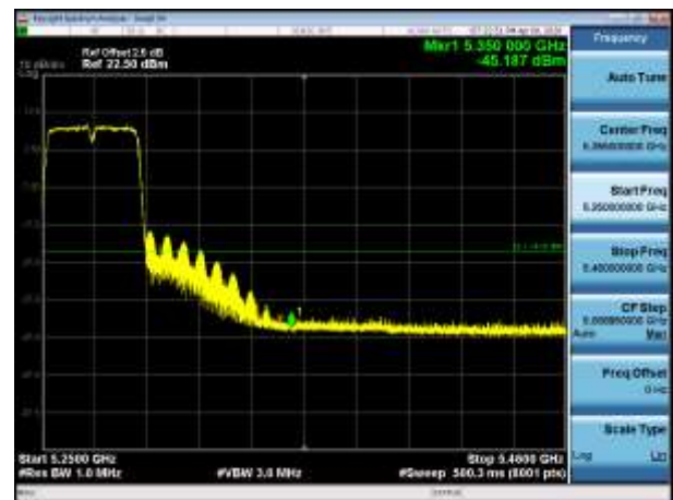
5270MHz PK
