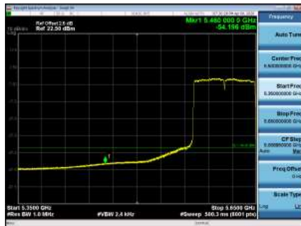
5610MHz AV
