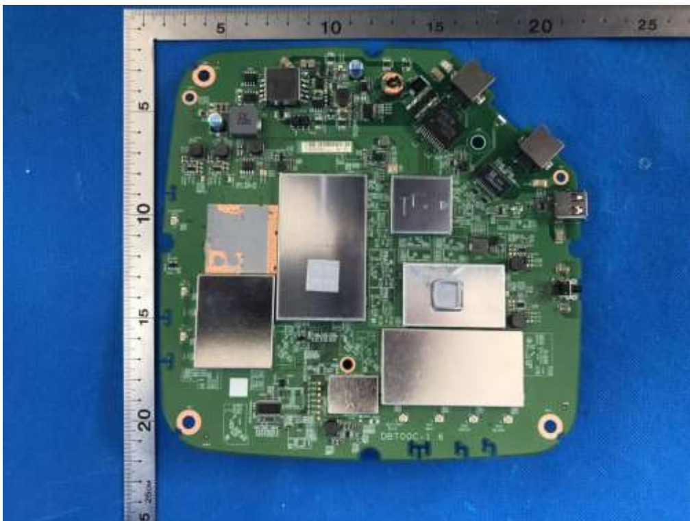
(4) EUT Photo(AP460C)
