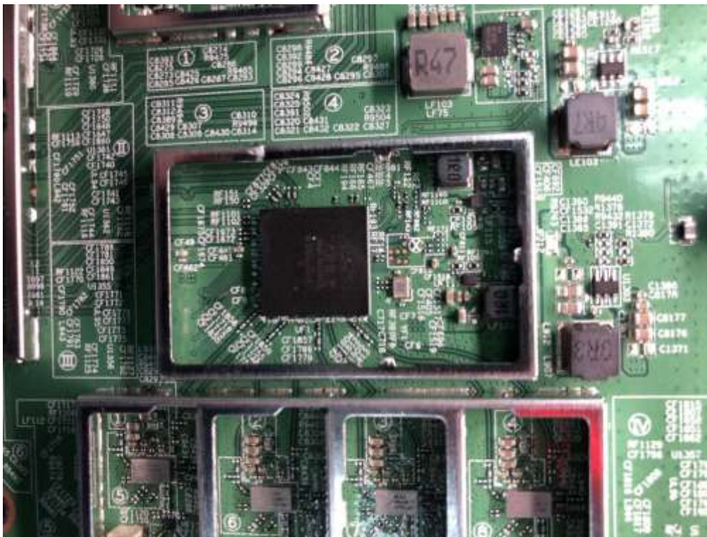
(10) EUT Photo(AP460C)
