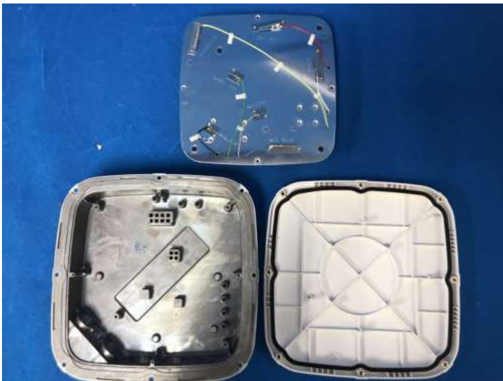
(2) EUT Photo(AP460C)
