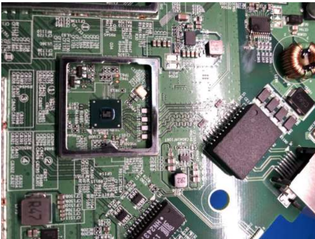
(6) EUT Photo(AP460C)
