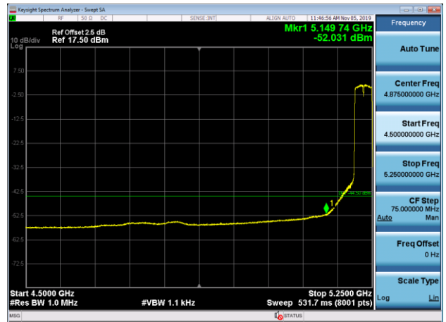
5230MHz AV
