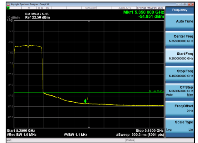
5270MHz AV
