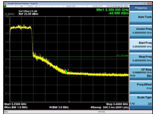
5270MHz PK
