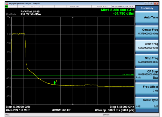
5300MHz AV
