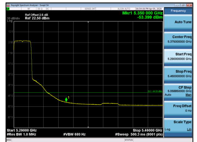
5300MHz AV
