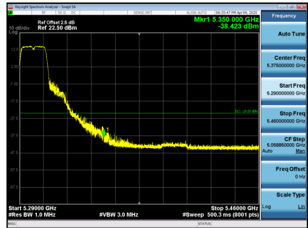
5300MHz PK
