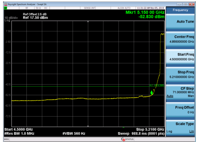
5200MHz AV
