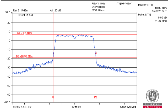
8802.11ac (VHT40)_Chain 1 / CH102
